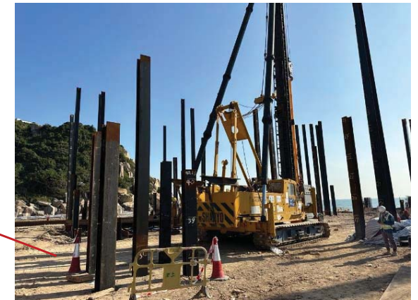
地基打樁施工
